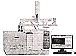
GC-MS
