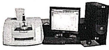
IR Spectroscopy
